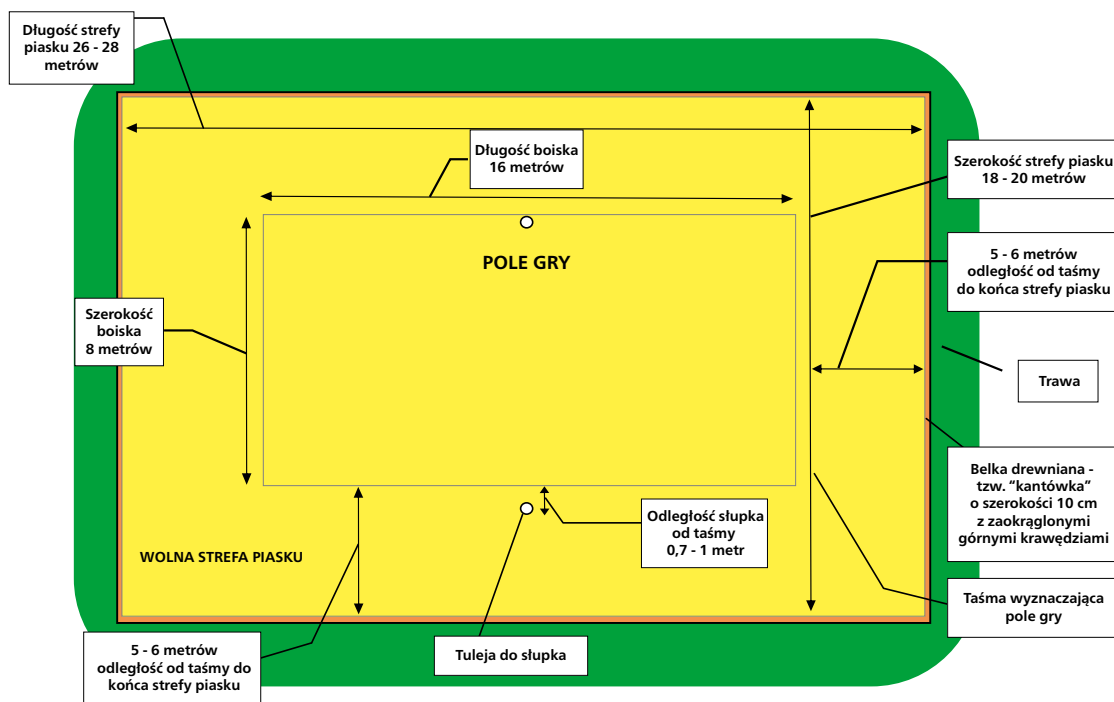
RYСУNEK 4. WIDOK BOISKA DO SIATKÓWKI PLAŻOWEJ WRAZ Z BEZPOŚREDNIM OTOCZENIEM
