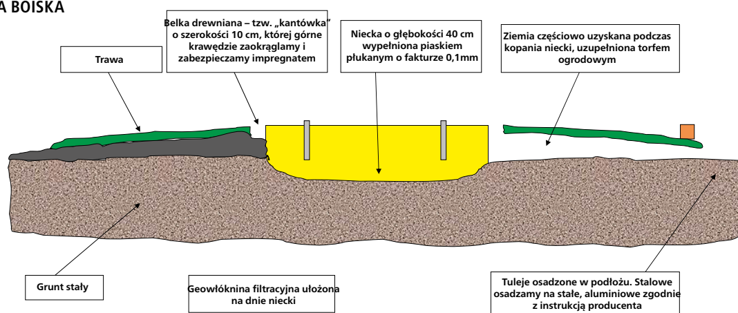
RYSUNEK 5. BUDOWA BOISKA
